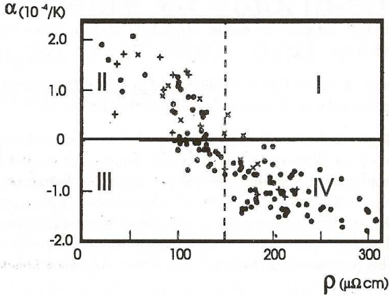
FIG. 1: Corrélation de Mooij à température ambiante pour des alliages massifs (+), des alliages en films minces (●) et des alliages amorphes (×), d'après [6].
