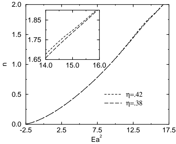
FIG. 8: La densité d'électrons pour des puits de potentiel de paramètre Va^2 = 1.4\hbar^2/(2m) et divers facteurs de remplissage \eta . Encart : vue détaillée dans le régime pseudo-gap.
