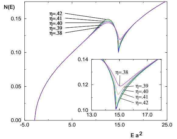
FIG. 6: Densité d'états pour des puits de potentiel de paramètre Va^2 = 1.4\hbar^2/(2m) et divers facteurs de remplissage \eta . Encart : vue détaillée dans le pseudo-gap.
