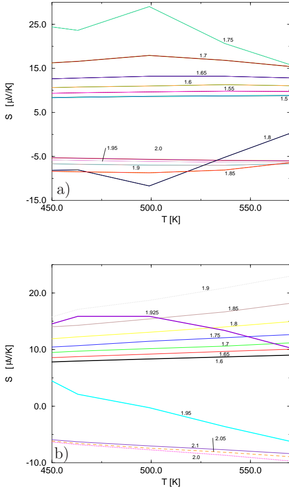
FIG. 15: Dépendance en température du pouvoir thermoélectrique pour a) Va^2 = 1.4\hbar^2/(2m) , et b) Va^2 = 1.9\hbar^2/(2m) .
