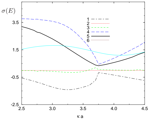
FIG. 11: Contributions à la conductivité pour des puits de potentiel de paramètre Va^2 = 1.9\hbar^2/(2m) et \eta = .42 . 1 : contribution vertex de X_1 , 2 : contribution vertex de X_4 , 3 : contributions vertex ++ et --, 4 : contribution de la fonction spectrale, 5 : conductivité totale et 6 : résultat de Ziman.
