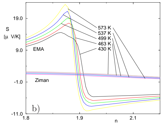
FIG. 14: Dépendance dans le taux de porteurs du pouvoir thermoélectrique pour a) Va^2 = 1.4\hbar^2/(2m) , et b) Va^2 = 1.9\hbar^2/(2m) .
